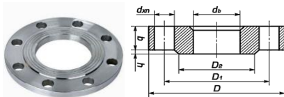
Фланец ГОСТ Ру10
