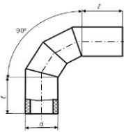
відвід 90° двосекційний
