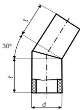
відвід 30° одностикової
