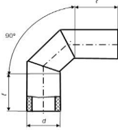
відвід 90° односекційний
