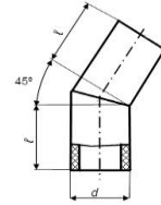
відвід 45° одностикової
