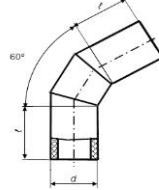
відвід 60° односекційний
